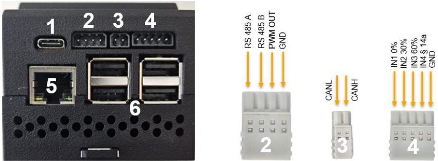
Abbildung 2: Anschlussmöglichkeiten Unterseite Primus
