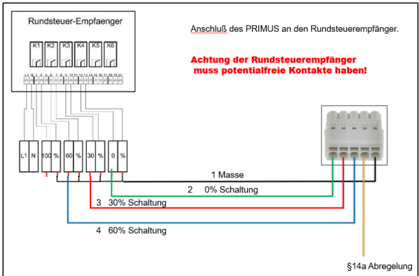
Abbildung 3: Anschluss an den Rundsteuerempfänger
