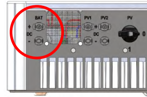
Abb. 28: Anschluss BAT (DC)
