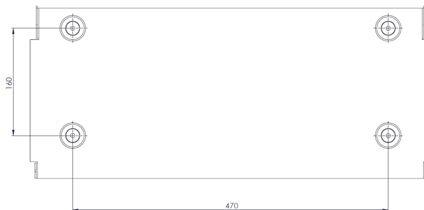
Abb. 8: Bohrungsmaße
