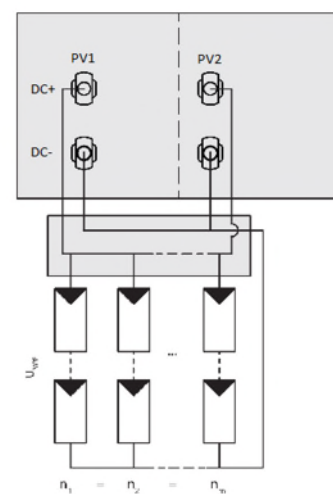
Abb. 23: Parallele Eingangsbeschaltung für ein oder mehrere Modulstränge.
