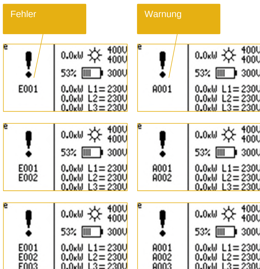
Abb. 55: Fehler und Warnungen in der Displayanzeige
