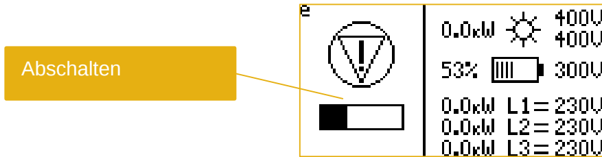
Abb. 53: Laufbalken beim herunterfahren
