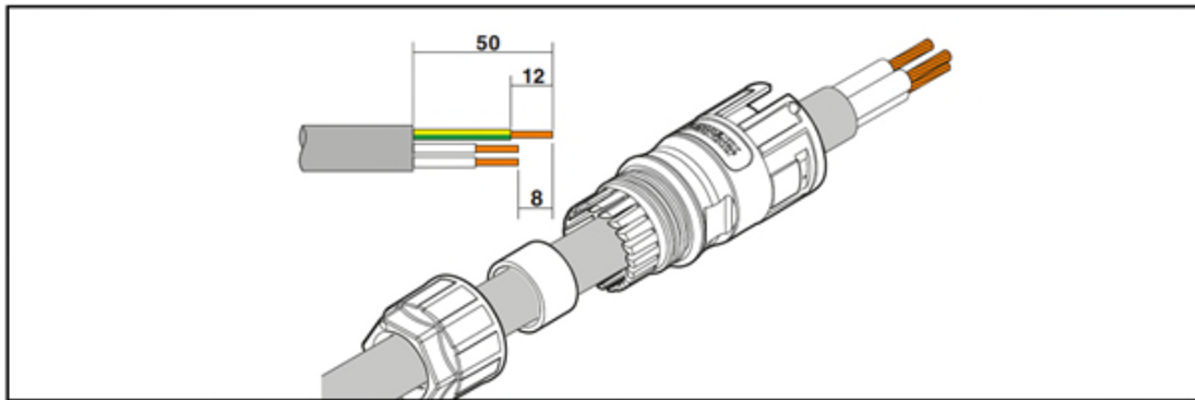
Abb. 13: Maße Abisolierung der Kabel
