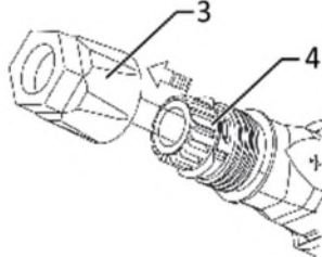
Abb. 25: Einsatz in Hülse schieben
