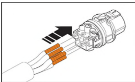
Abb. 14: Adern auflegen
