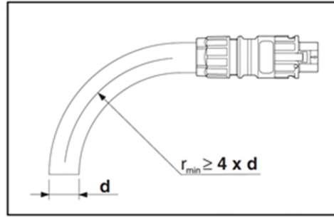
Abb. 19: Mindestbiegeradius
