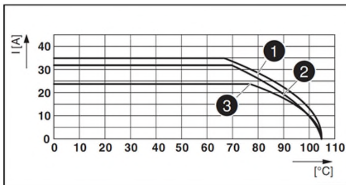
Abb. 20: Maximalströme und Derating gemäß verwendeter Kabelquerschnitte.
