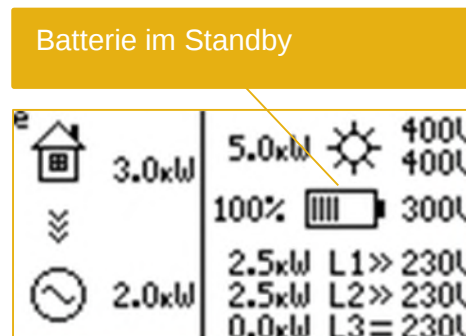
Abb. 39: Batterie im Standby Modus
