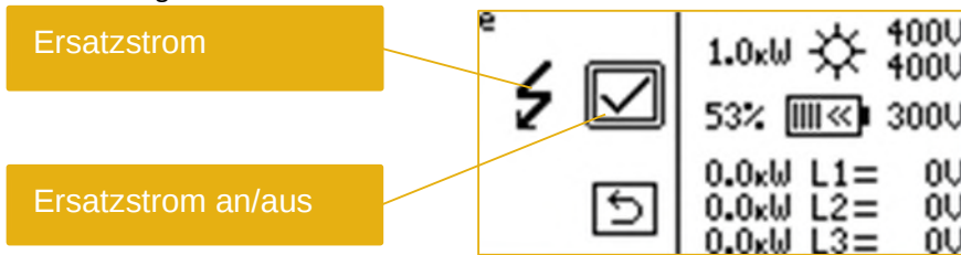
Abb. 50: Insel- oder Ersatzstrom Freischaltung
