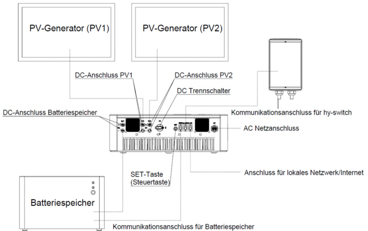
Abb. 11: Übersicht der Anschlüsse
