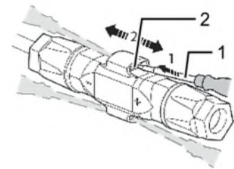
Abb. 62: Steckverbinder abstecken
