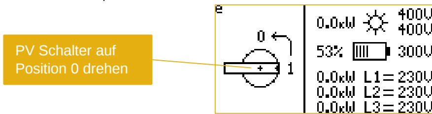
Abb. 54: PV Schalter ausschalten
