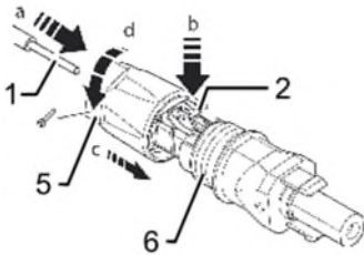
Abb. 24: Adern einfügen
