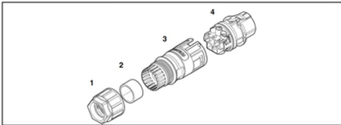
Abb. 12: AC Stecker
