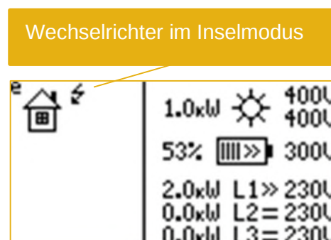
Abb. 40: Wechselrichter im Inselnetzbetrieb
